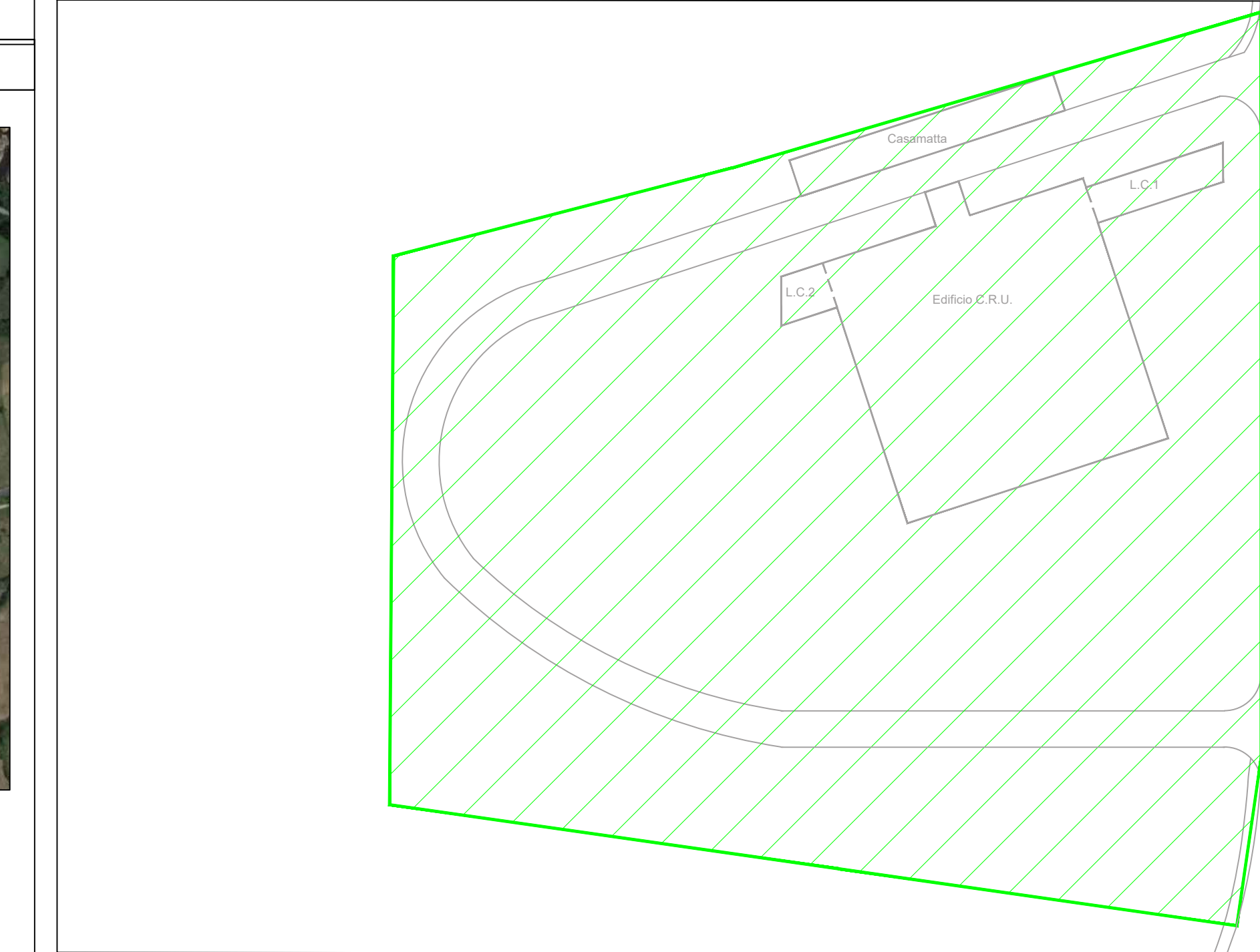
AREA DI BONIFICA SUPERFICIALE E PROFONDA secondo il D.Lgs. 81/08 e successiva Legge 177/2012.
