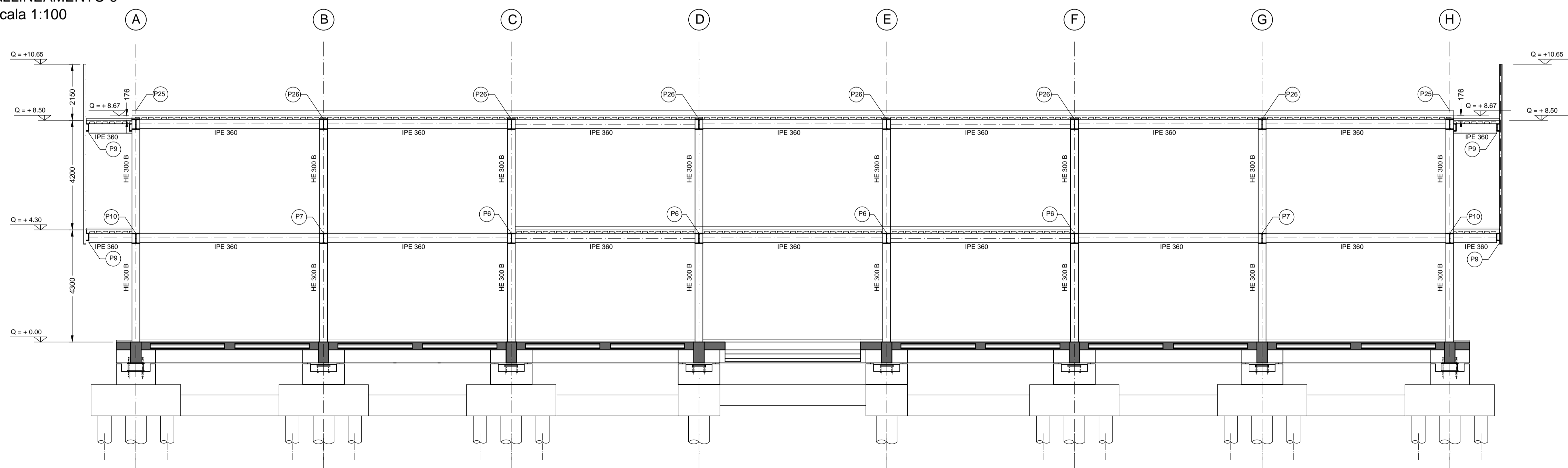
SEZIONE ALLINEAMENTO 6 scala 1:100
