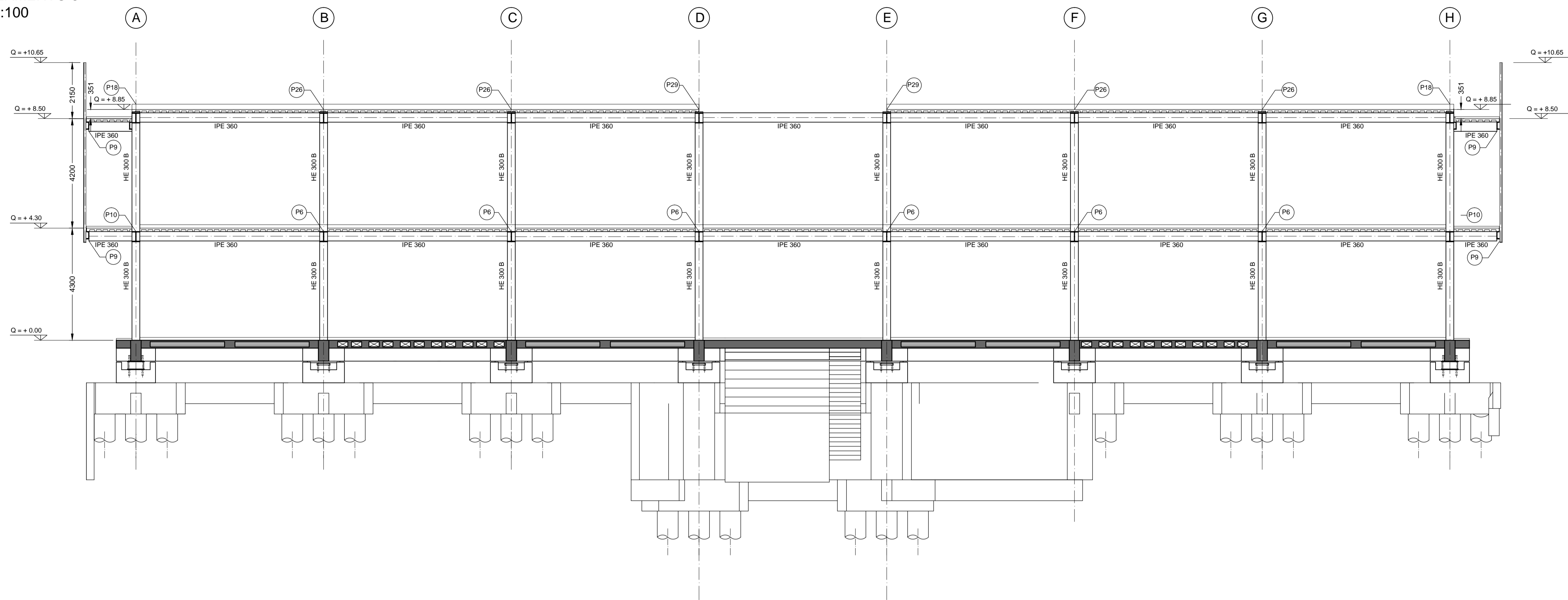
SEZIONE ALLINEAMENTO 5 scala 1:100
